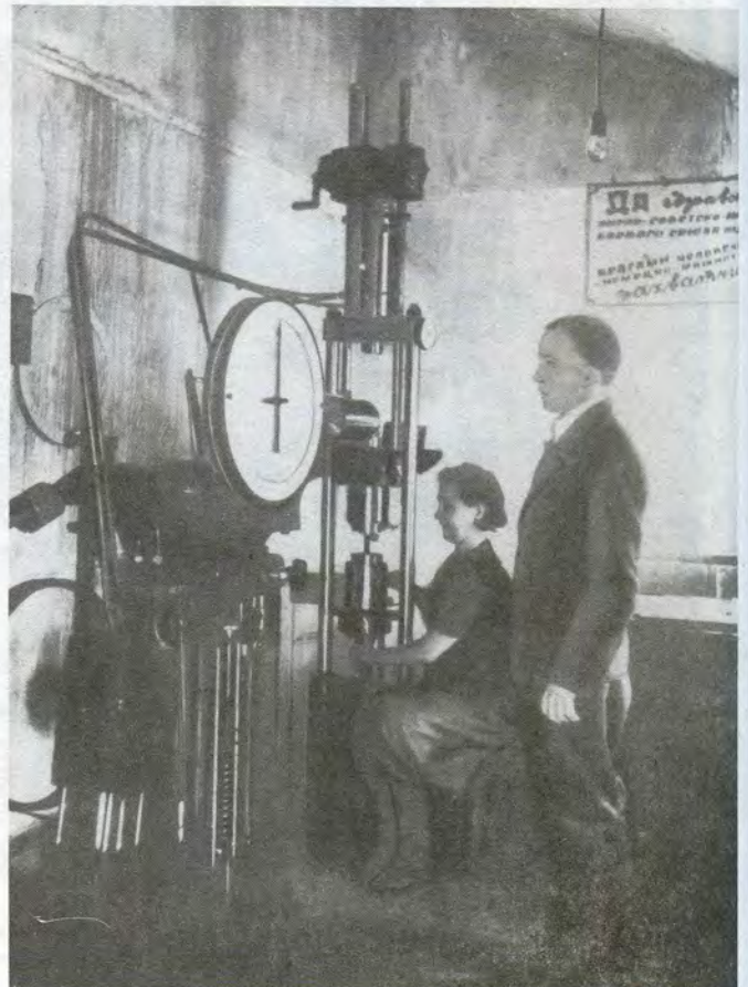
Испытания авиационной фанеры в лаборатории Мантуровского фанерного завода. 1944 г. (из фондов Государственного архива Костромской области)
